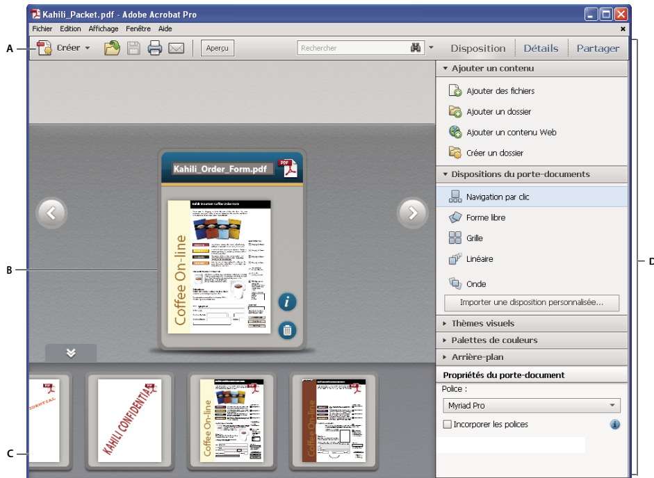
Porte-documents PDF en mode de disposition Navigation par clic mise en page dans Acrobat Pro A. Barre d'outils des porte-documents PDF B. Carte représentant le fichier composant C. Fichiers et dossiers composants dans le mini-navigateur D. Panneau Disposition pour personnaliser l'aspect
