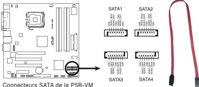
Connecteurs SATA de la P5B-VM
